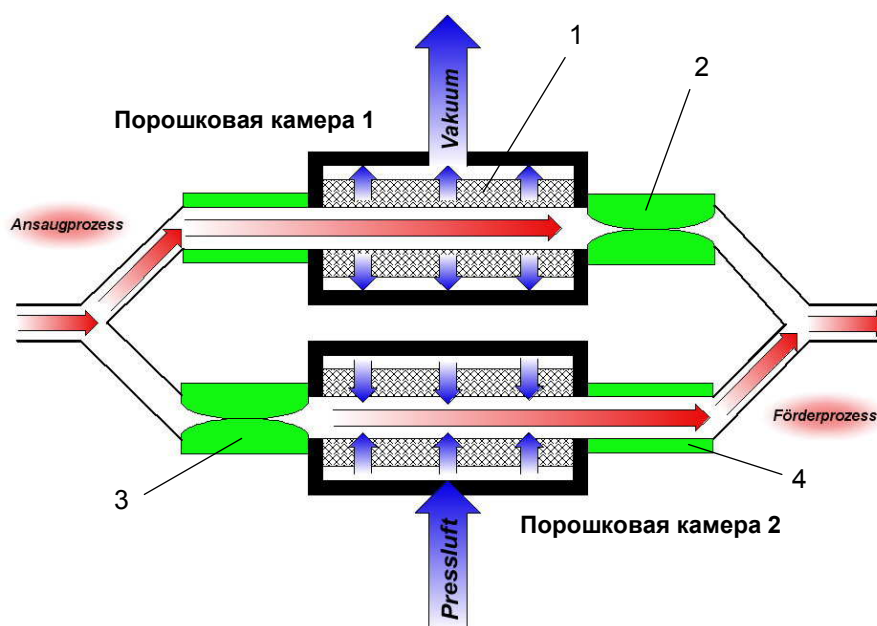
Принцип работы порошкового насоса OptiFeed PP06
